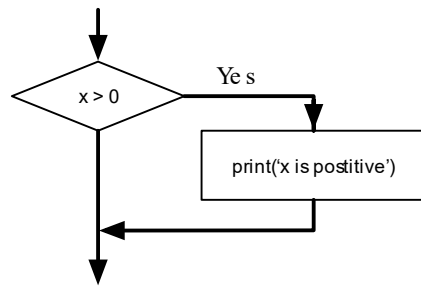
If Logic
